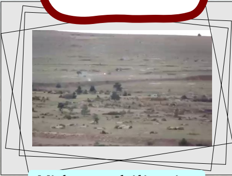
Video stabilisation
